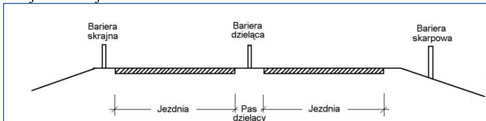
Rys. 2. Schemat odcinka bariery z lin stalowych
