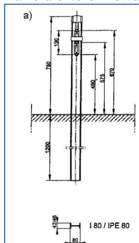
Rys. 4. Przykłady ustawienia słupków barier linowych
