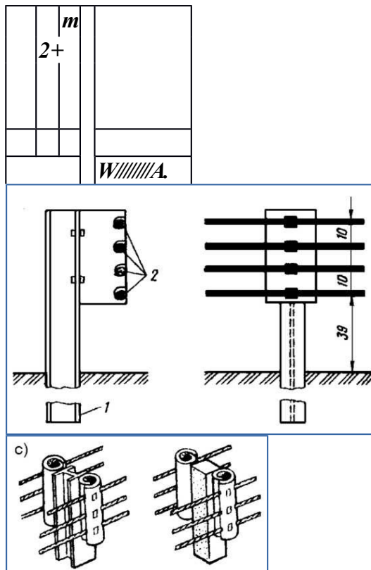
Rys. 4. Przykłady ustawienia słupków barier linowych
