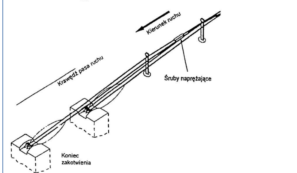
Rys. 10. Przykład zakotwienia lin na odcinku początkowym bariery czterolinowej z dwoma blokami kotwiącymi
