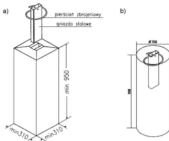
Rys. 9. Przykładowy schemat bariery czterolinowej
