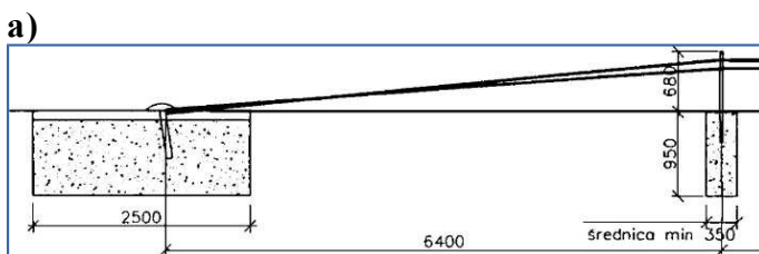
Rys. 6. Przykłady ukośnego odcinka początkowego bariery linowej a) Bariera trzylinowa, b) Bariera czterolinowa
