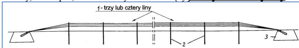
Rys. 3. Przykłady umocnienia lin do słupków
