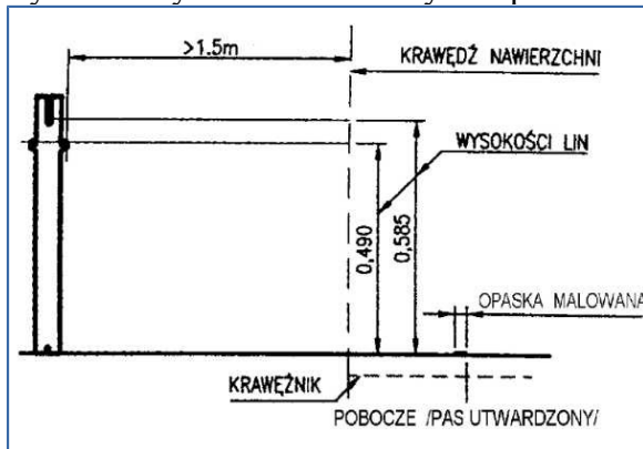
Rys. 1.3. Wysokość lin bariery nad poboczem i pasem dzielącym
